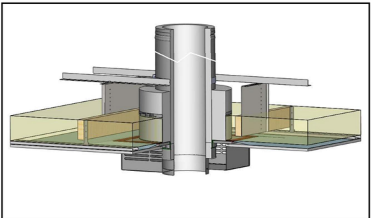
Figure 7b – Mise en œuvre des composants du procédé KIT ISOLETANCHE autour du conduit métallique
