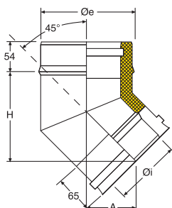
Coude 45°
