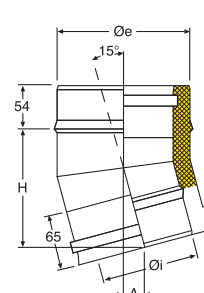
Coude 15°
