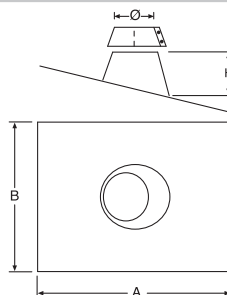
Solin incliné
