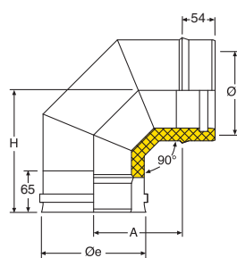
Coude 90°
