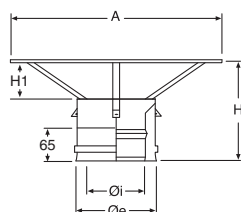
Chapeau chinois
