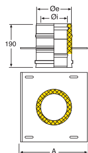
Plaque intermédiaire
