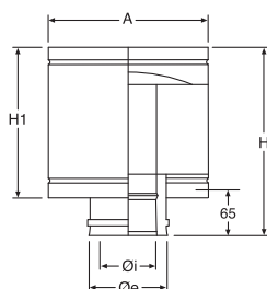
Terminal anti-intéférences
