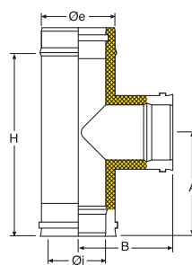
Té à 90°
