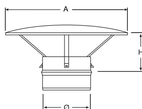
Chapeau chinois
