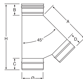
Té à 135°
