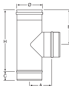
Té à 90°
