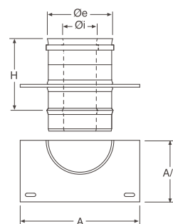
Plaque intermédiaire
