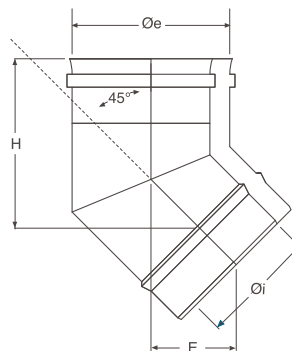
Coude 45°
