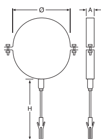
Collier mural de fixation
