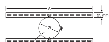
Collier de soutien avec cornières
