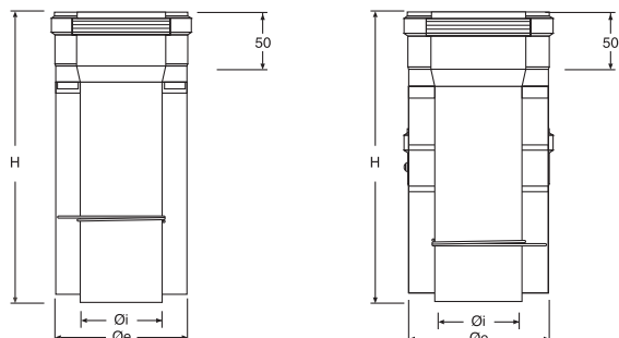
Longueur 2 m / 1 m / 0,5 m / 0,25 m
