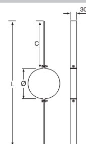
Collier boisseau
