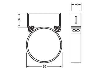
Collier mural non réglable
