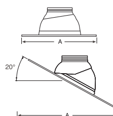
Solin 5°-18°
