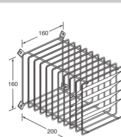
Panier de protection
